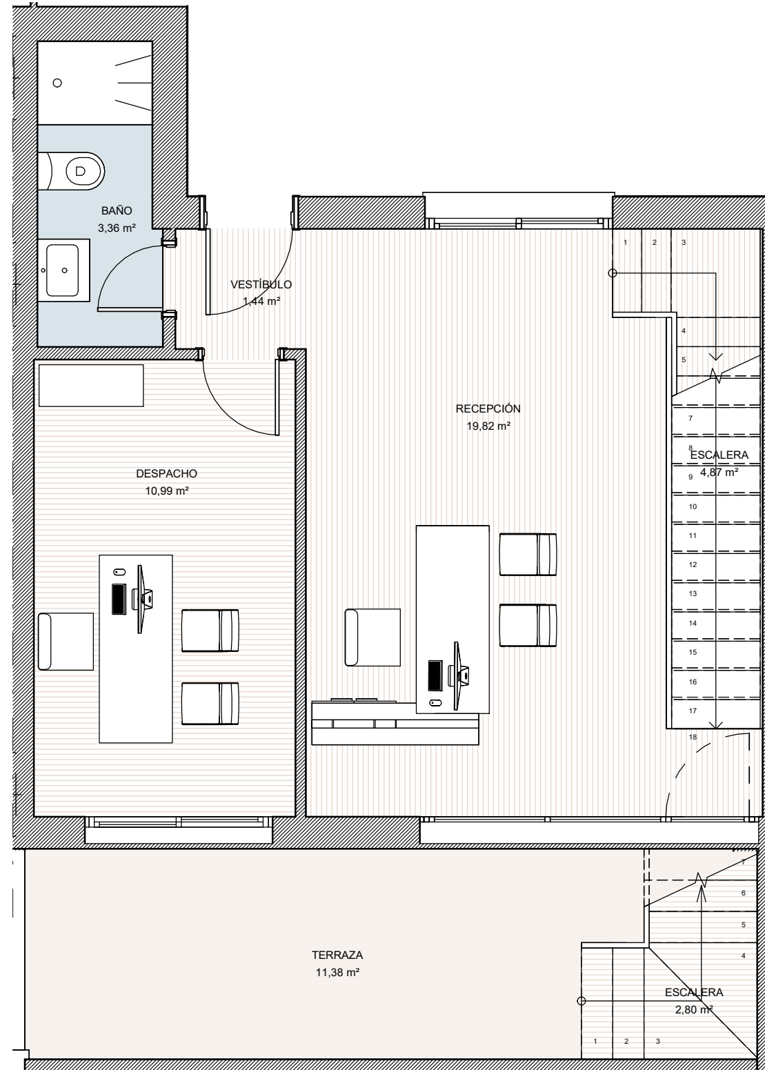
PLANTA BAJA
