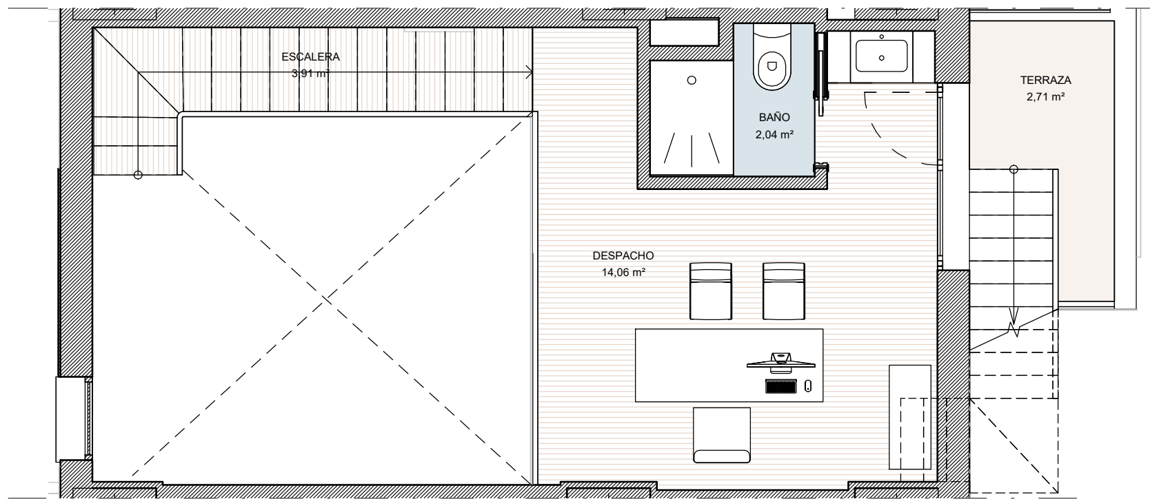
PLANTA PRIMERA
