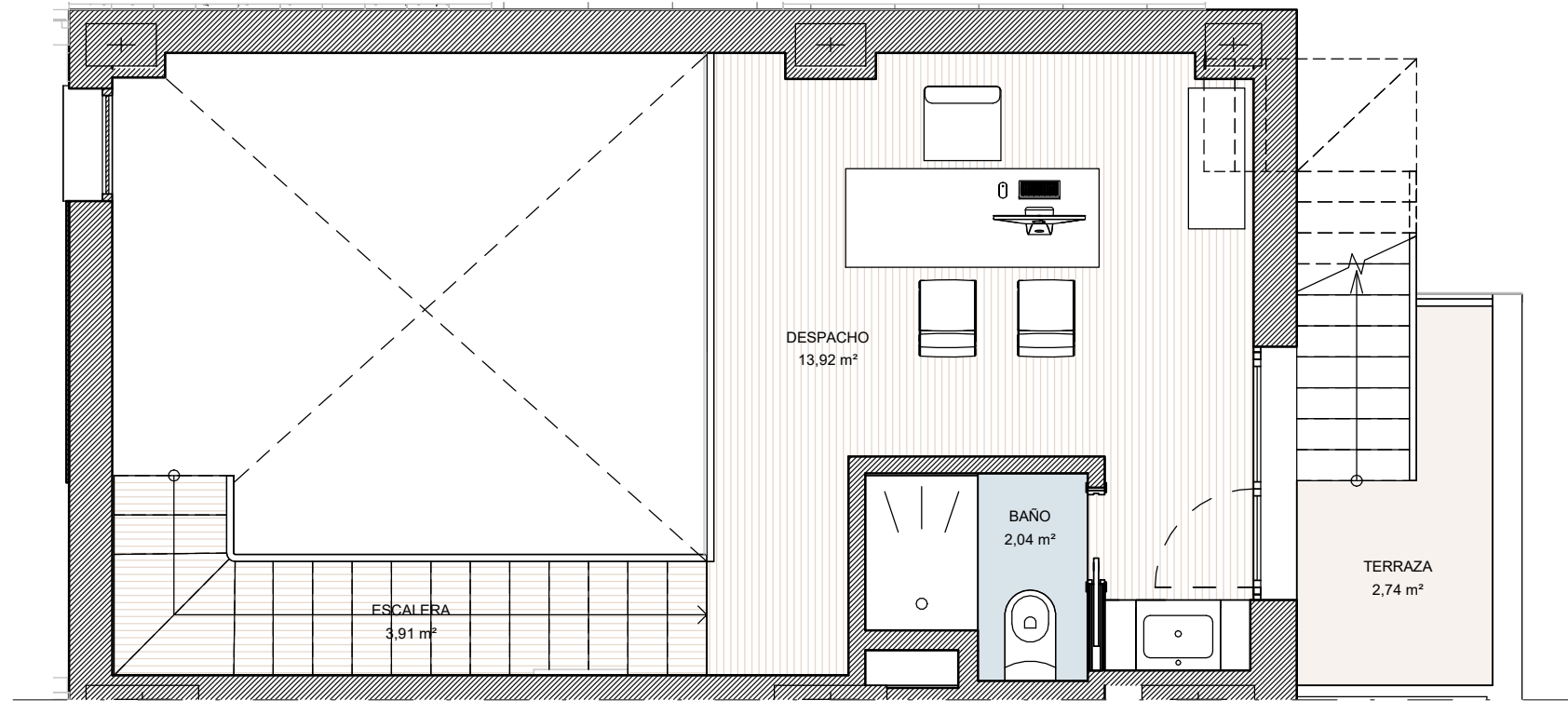
PLANTA PRIMERA
