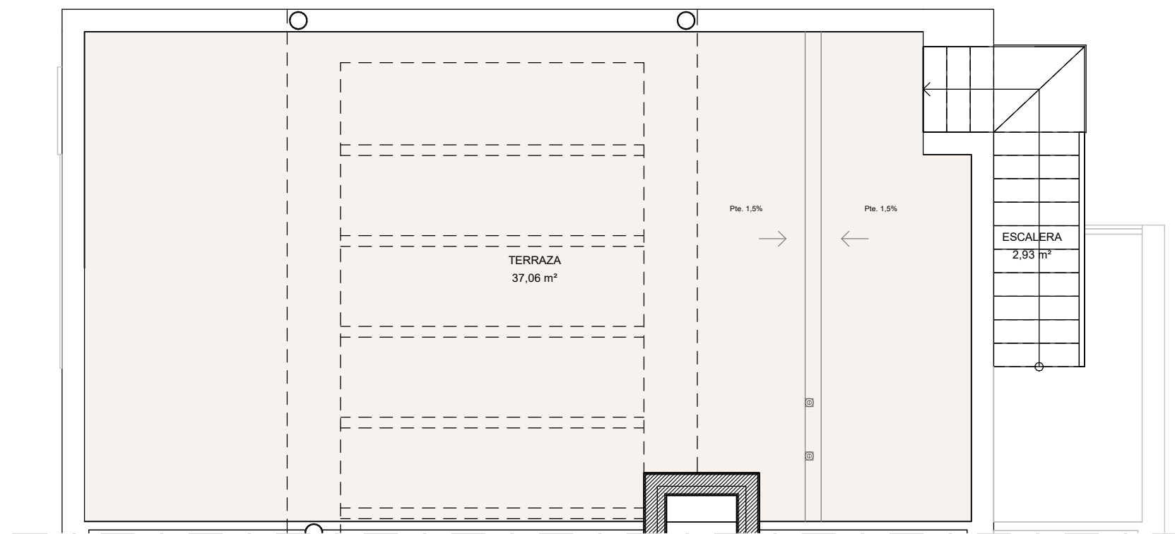
PLANTA CUBIERTA
