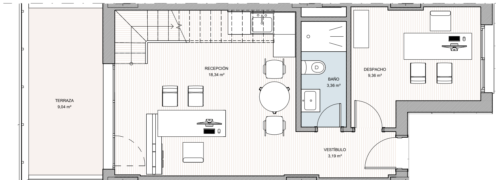
PLANTA BAJA
