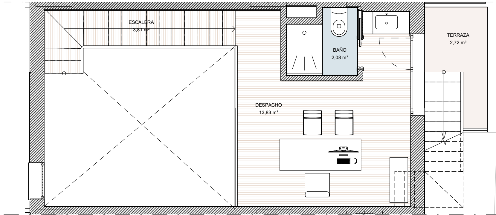
PLANTA PRIMERA
