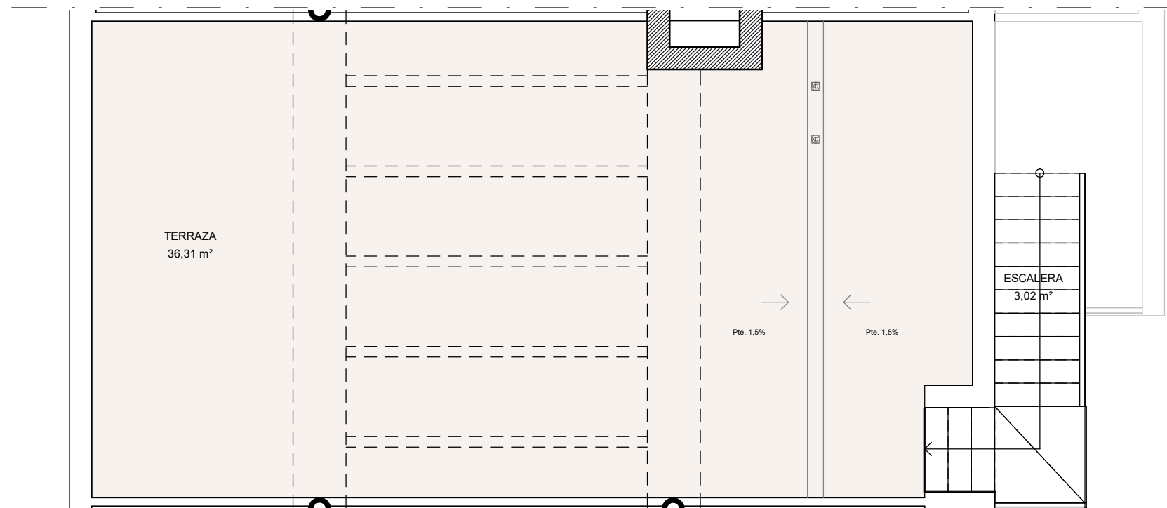
PLANTA CUBIERTA
