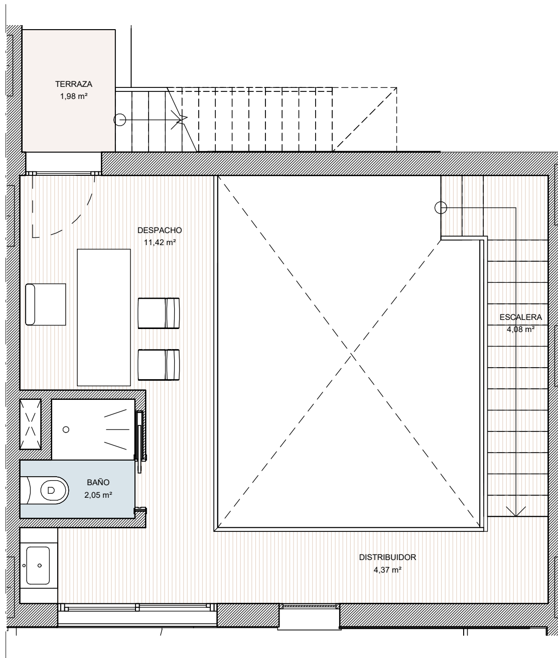
PLANTA PRIMERA
