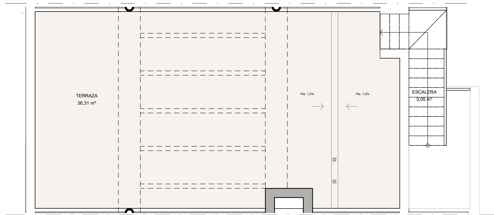
PLANTA CUBIERTA
