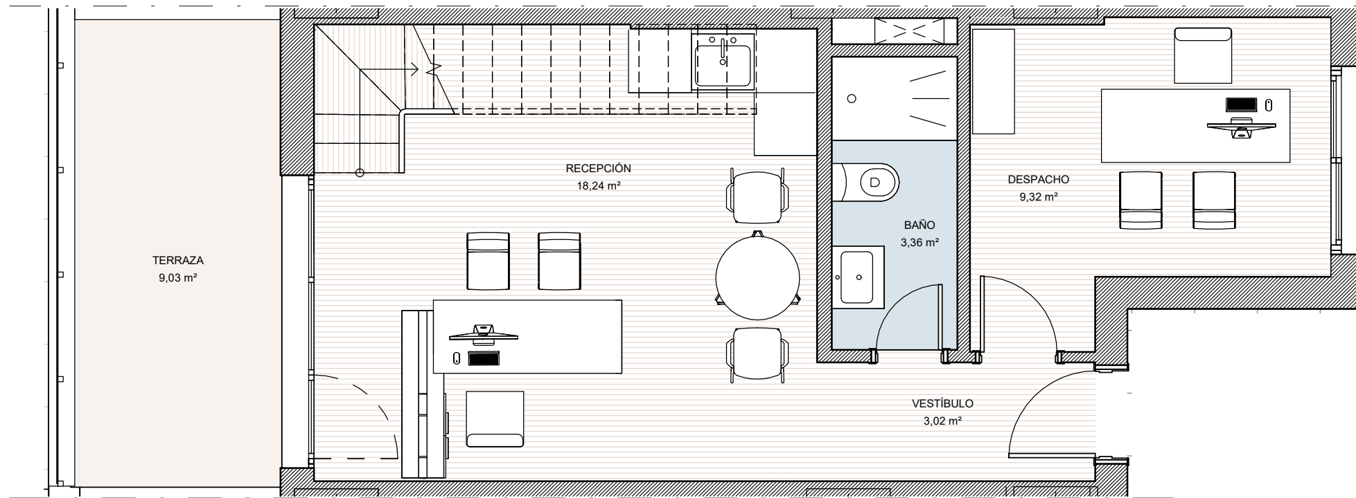
PLANTA BAJA
