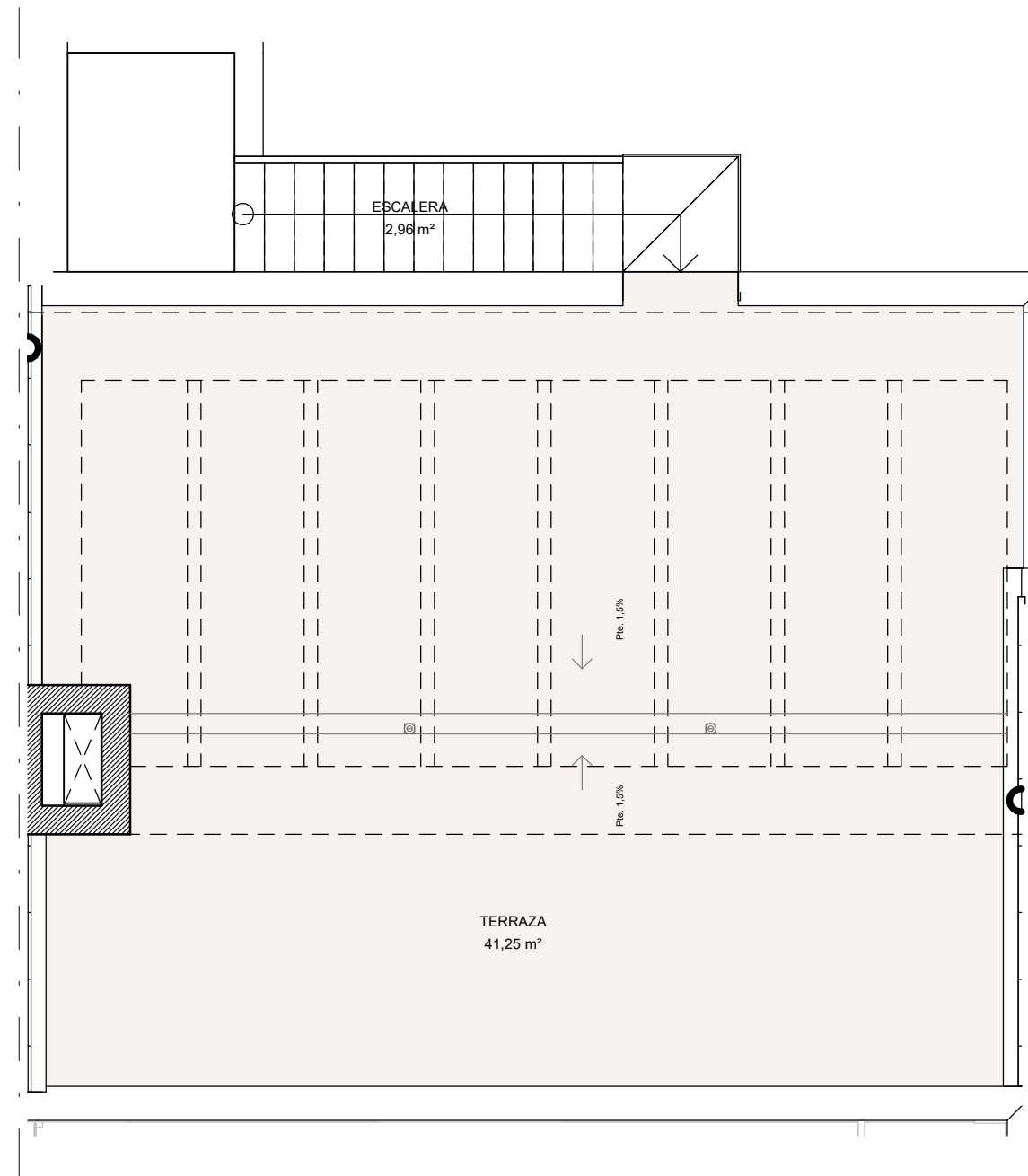
PLANTA CUBIERTA
