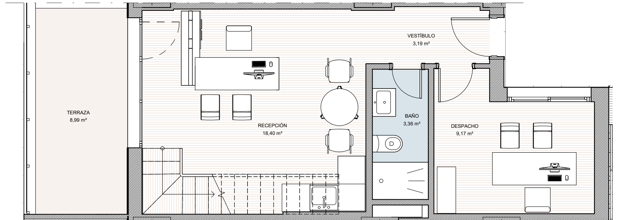
PLANTA BAJA
